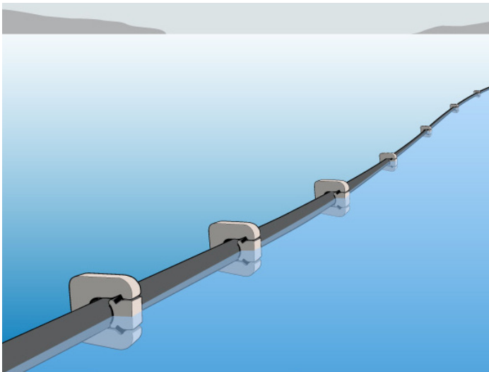
7. Ledningen fylls, under utläggningen, med luft så att den flyter på ytan. När viktningen är klar fylls ledningen med vatten...
